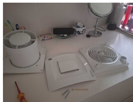
Fig. 6 Extractor S&P Silen dual 300 despiezado para empezar instalación.
